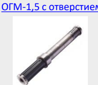
Вал шлицевой под усиленный подшипник 120х806 ОГМ-1,5 с отверстием
